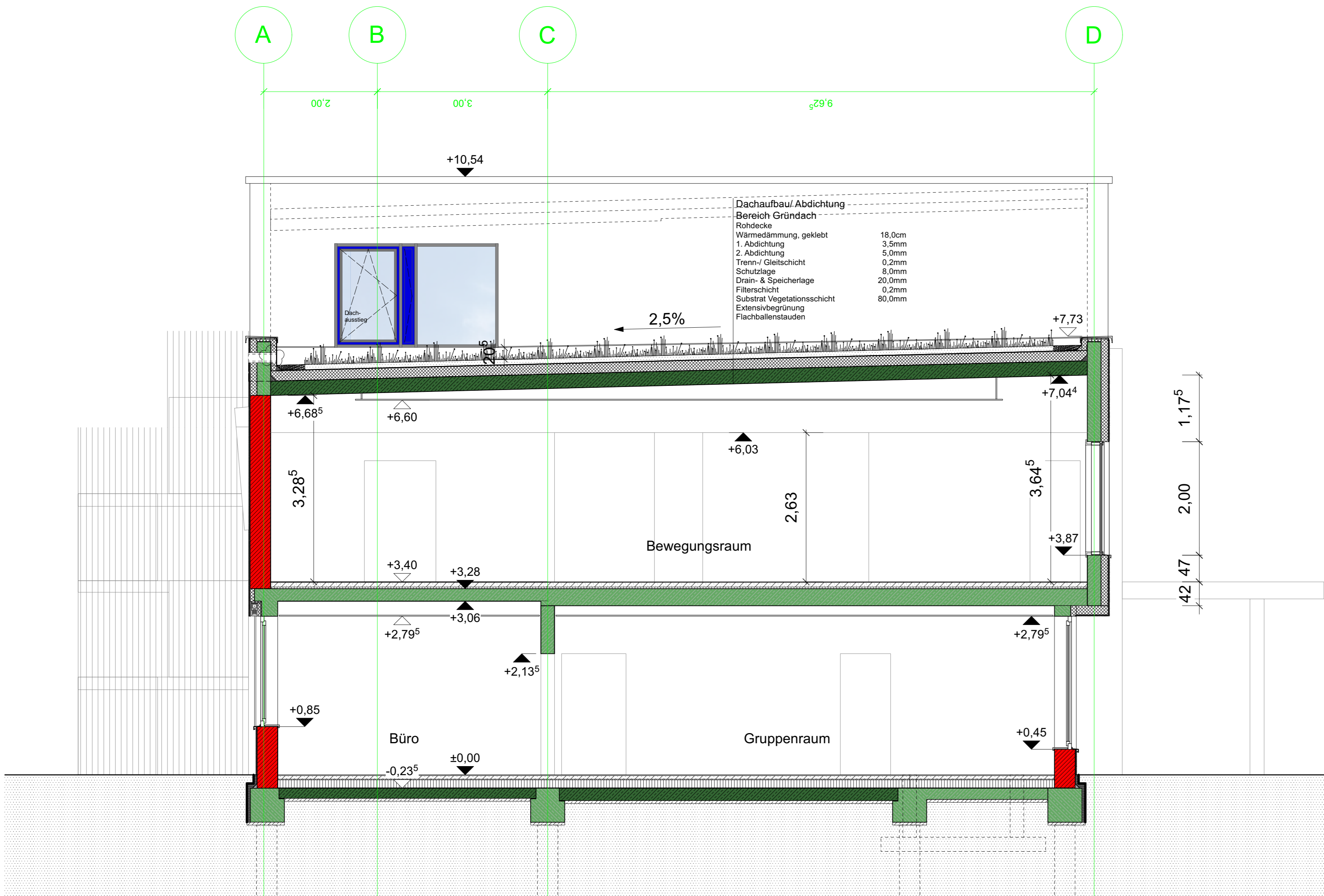
Schnitt E-E
