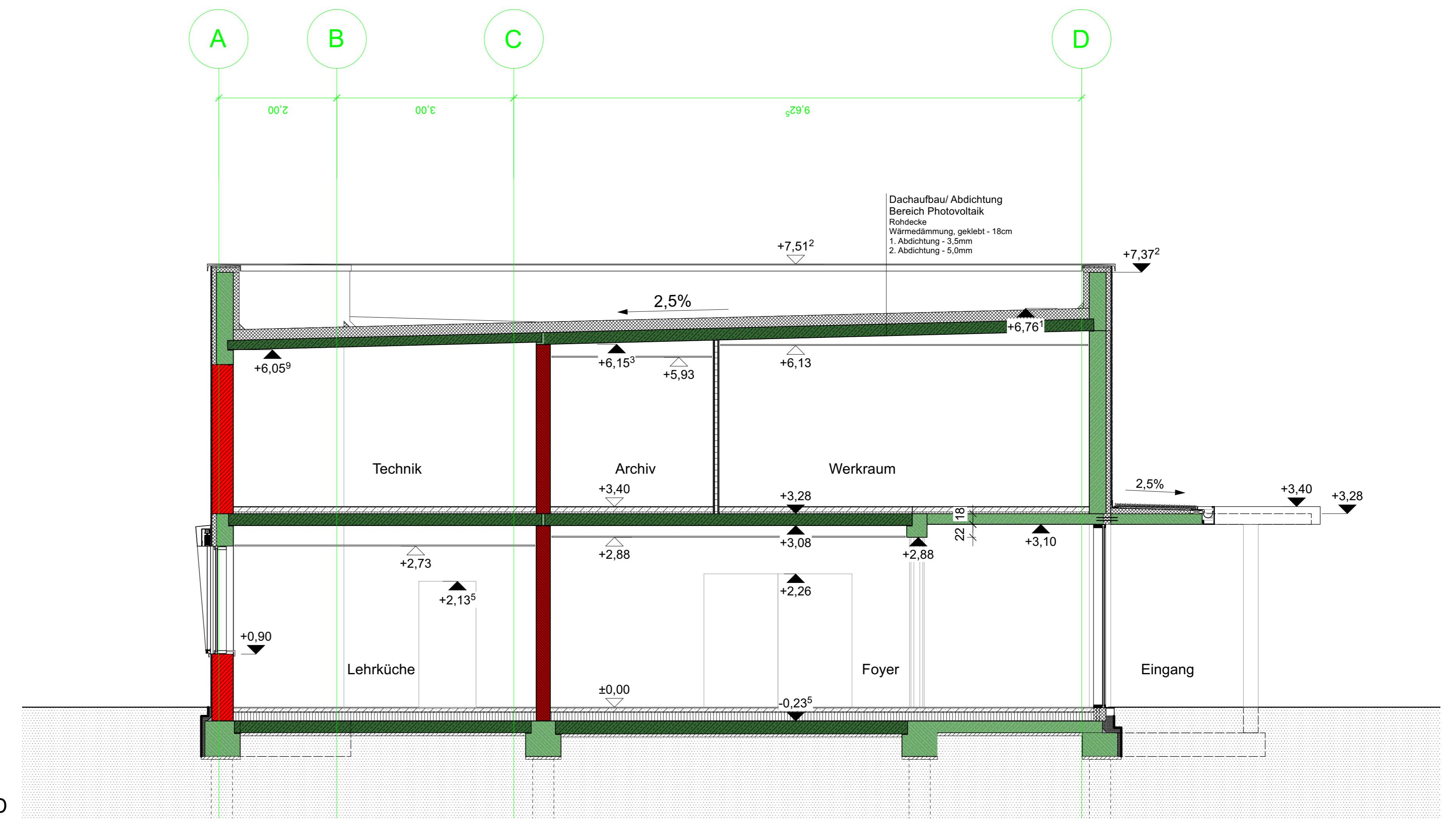
Schnitt D-D
