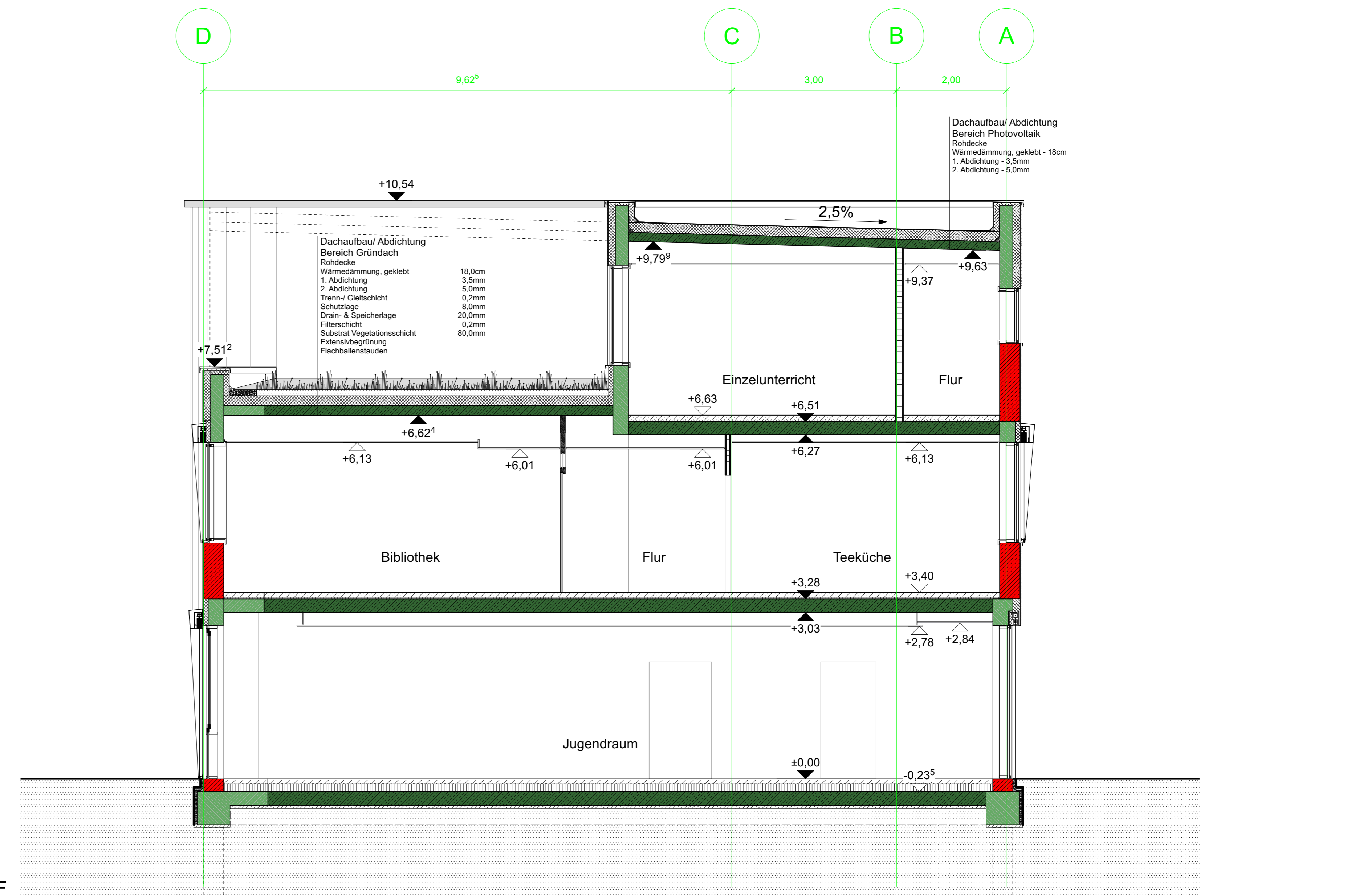
Schnitt F-F
