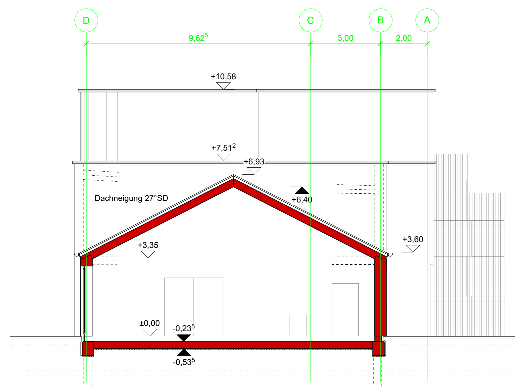
Schnitt C-C
