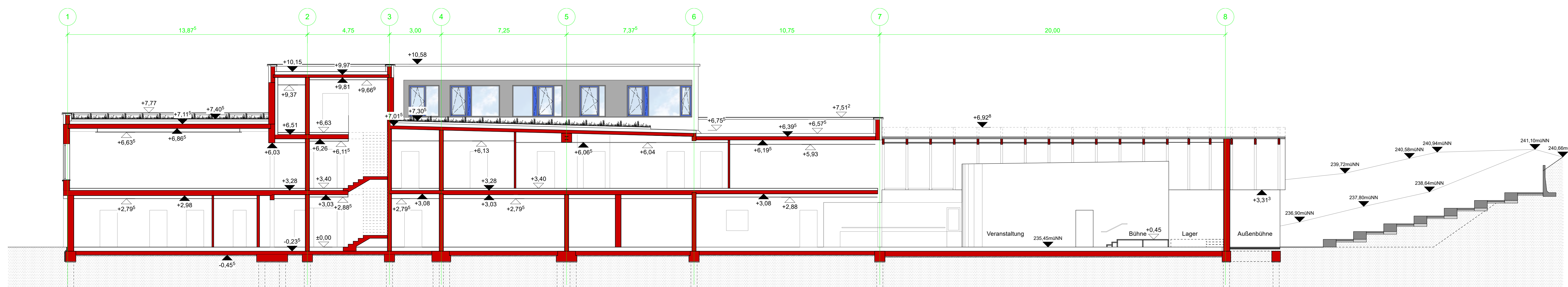
Schnitt A-A
