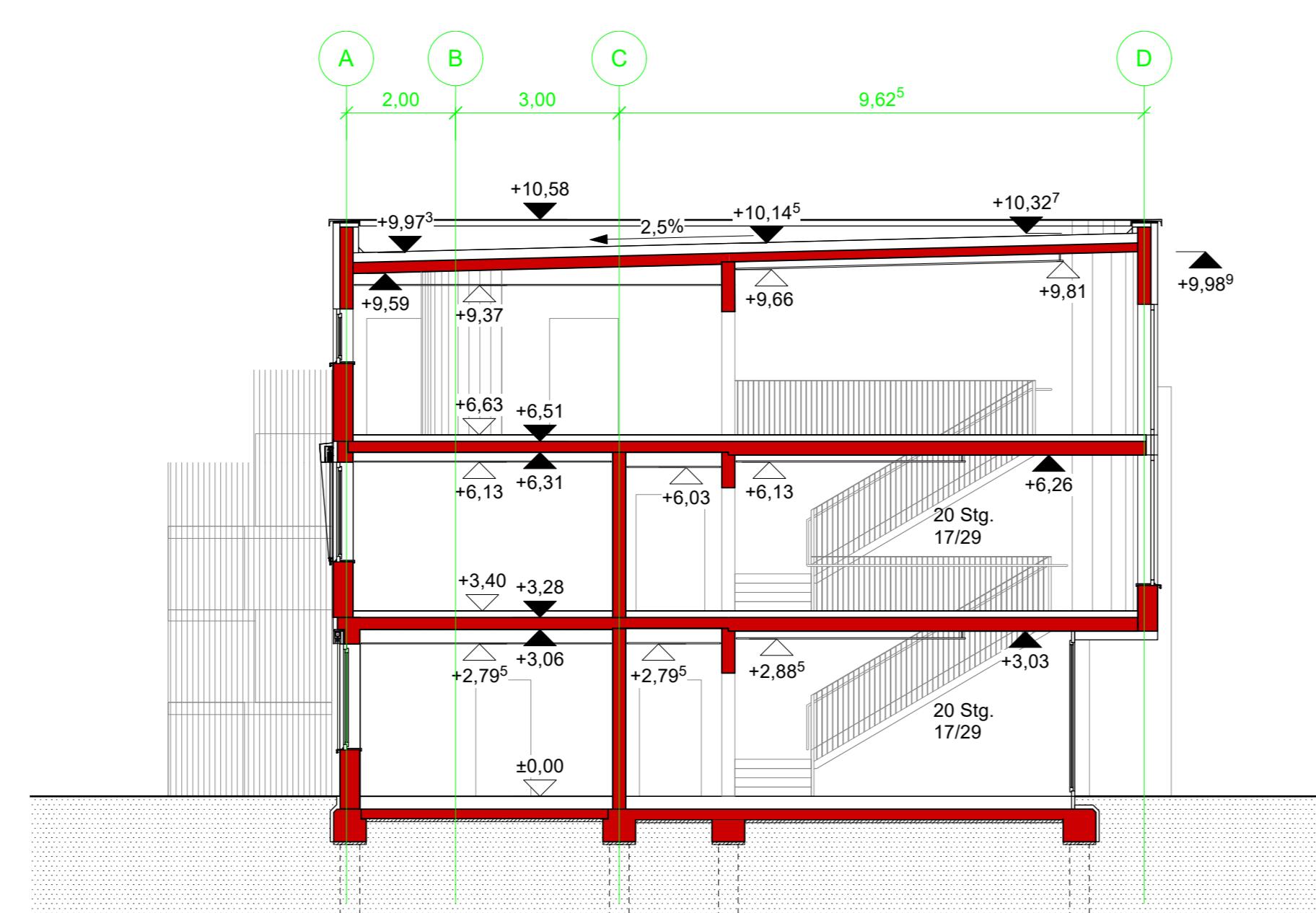
Schnitt B-B
