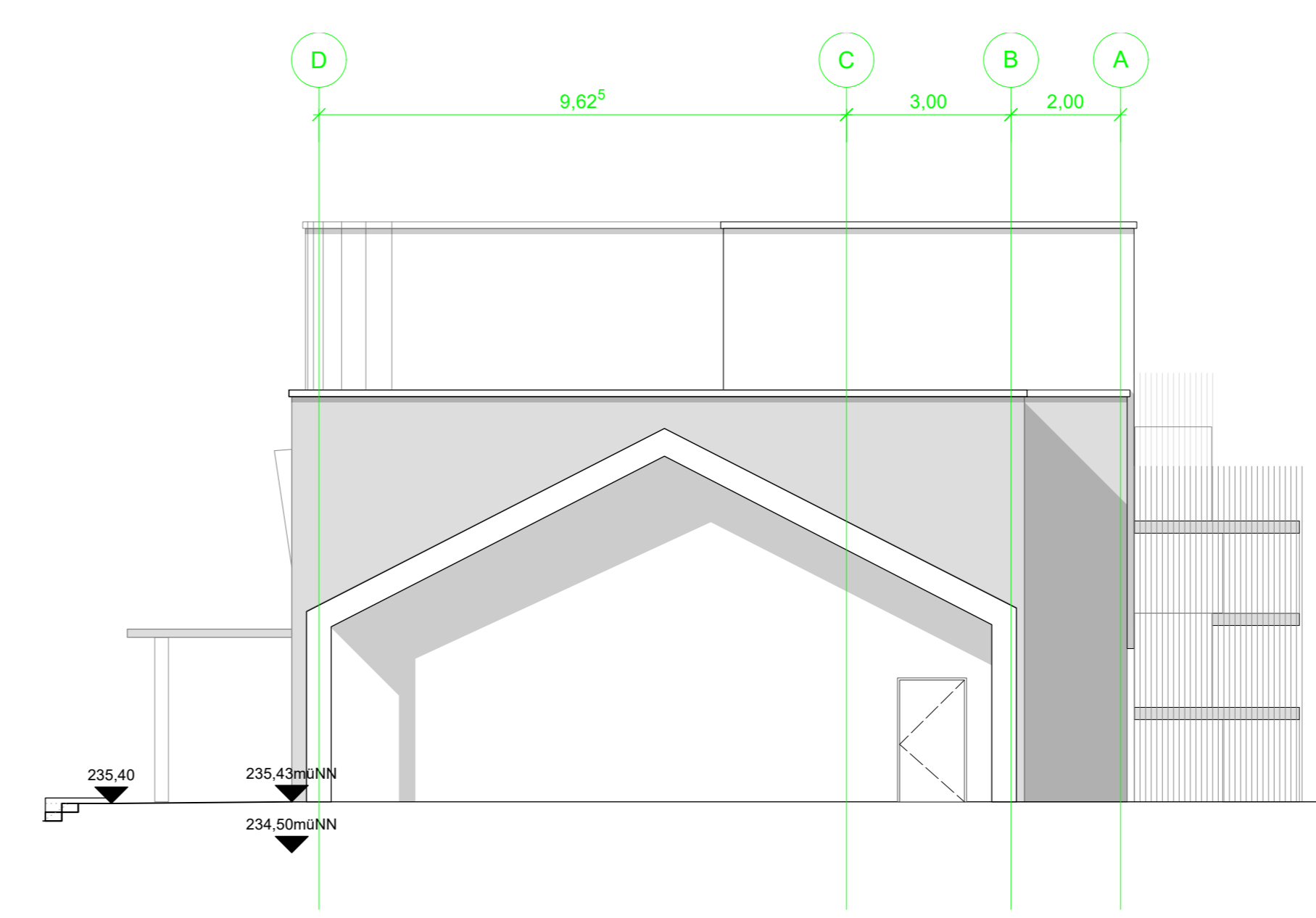
Südansicht
